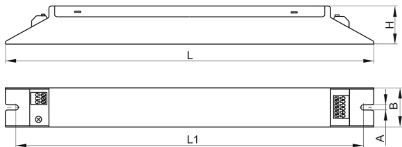
Рисунок 1. Габаритные и установочные размеры ЭПРА
